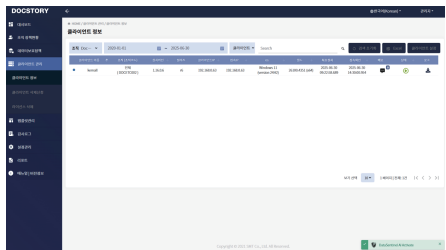
4. 클라이언트 정보
