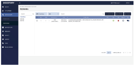
3. 데이터보호정책 (차단프로세스)
