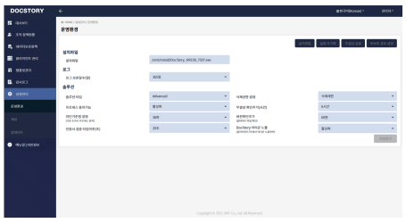
6. 설정관리
